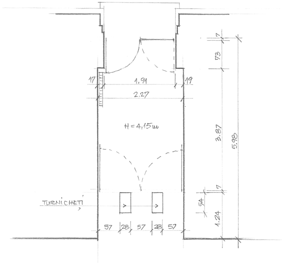
ACCES PRINCIPAL (B) ÎN PREZENT FUNCȚIONAL RELEVÉU SC. 1:50
